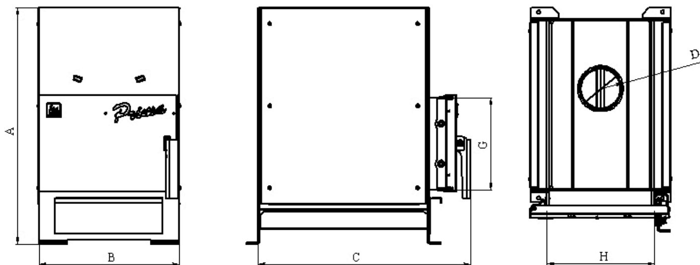
Рис. 1 Основные размеры печи PRIMA
