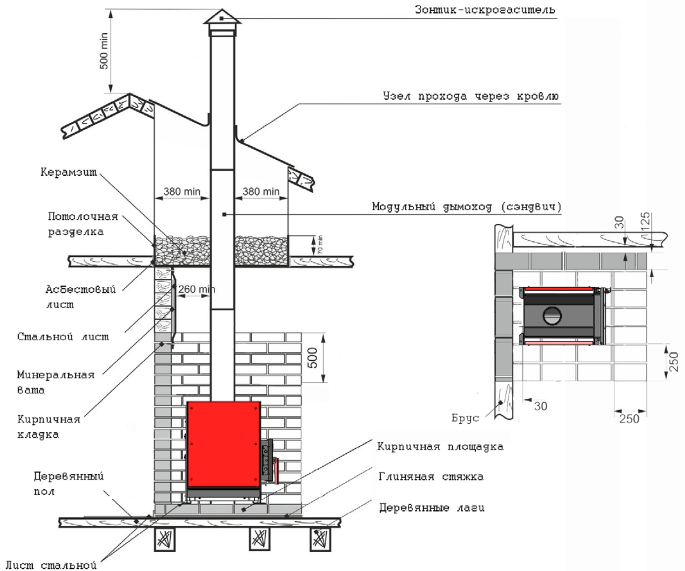
Рис. 3 Монтаж печи PRIMA
